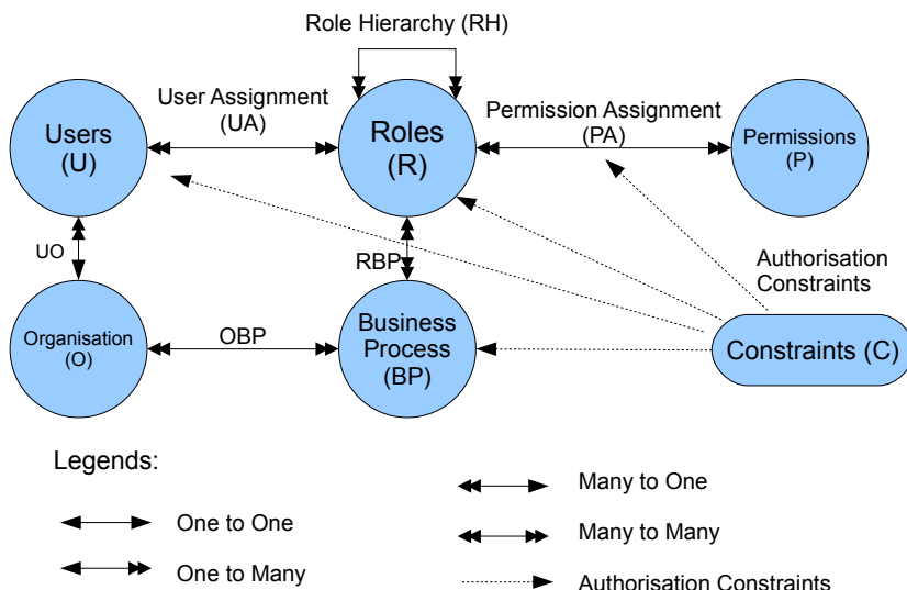
Fig. 4. BPEL4RBAC Model
